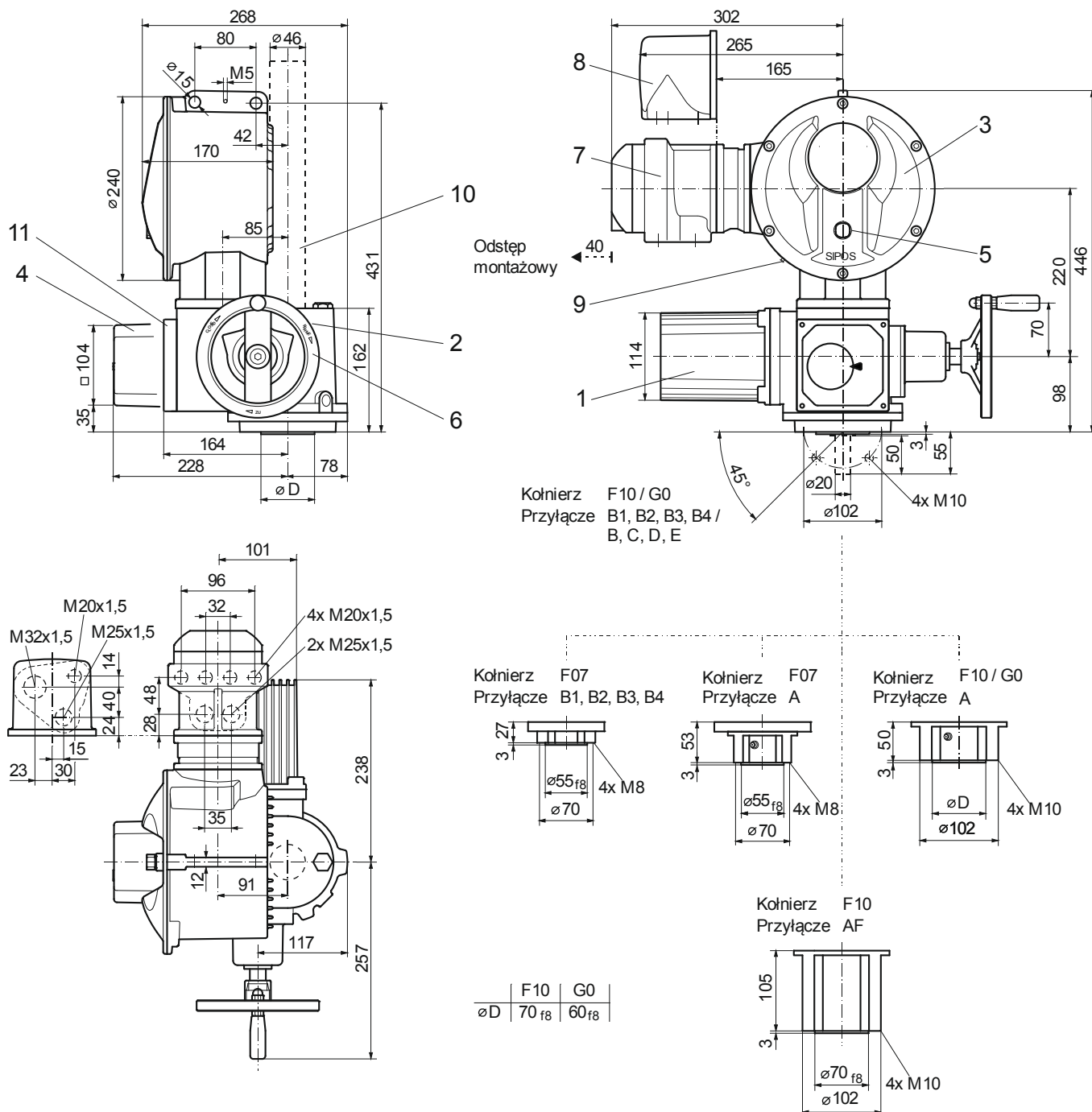
Rysunek wymiarowy 2SA701., 2SA702., 2SA731., 2SA732., 2SA751., 2SA752.
