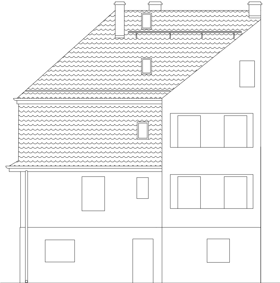
elewacja główna od ulicy Dąbrowskiego
