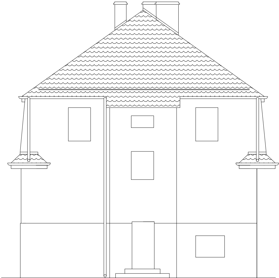
elewacja wejściowa od ul. Klonowej
